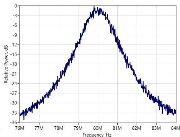
RF-line Spectrum
